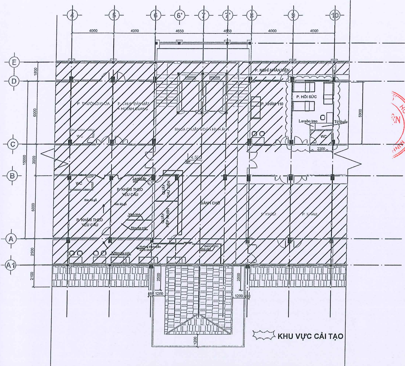
MẶT BẰNG CẢI TẠO PHÒNG KHÁM 112 TL:1/100
