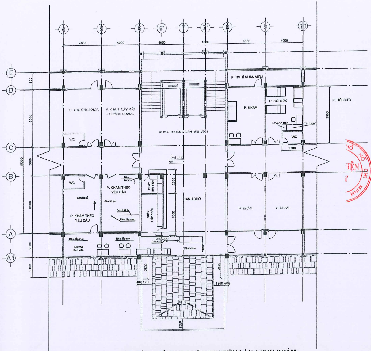
MẶT BẰNG CẢI TẠO QUẦY THU TIỀN LẦU 1 KHU KHÁM VÀ ĐIỀU TRỊ TRONG NGÀY TL:1/100
