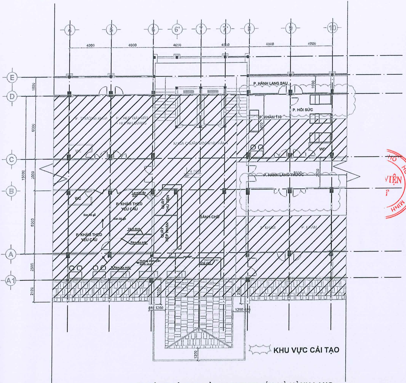
MẶT BẰNG CẢI TẠO HÀNH LANG TRƯỚC VÀ HÀNH LANG SAU PHÒNG 110 VÀ PHÒNG 112 TL:1/100
