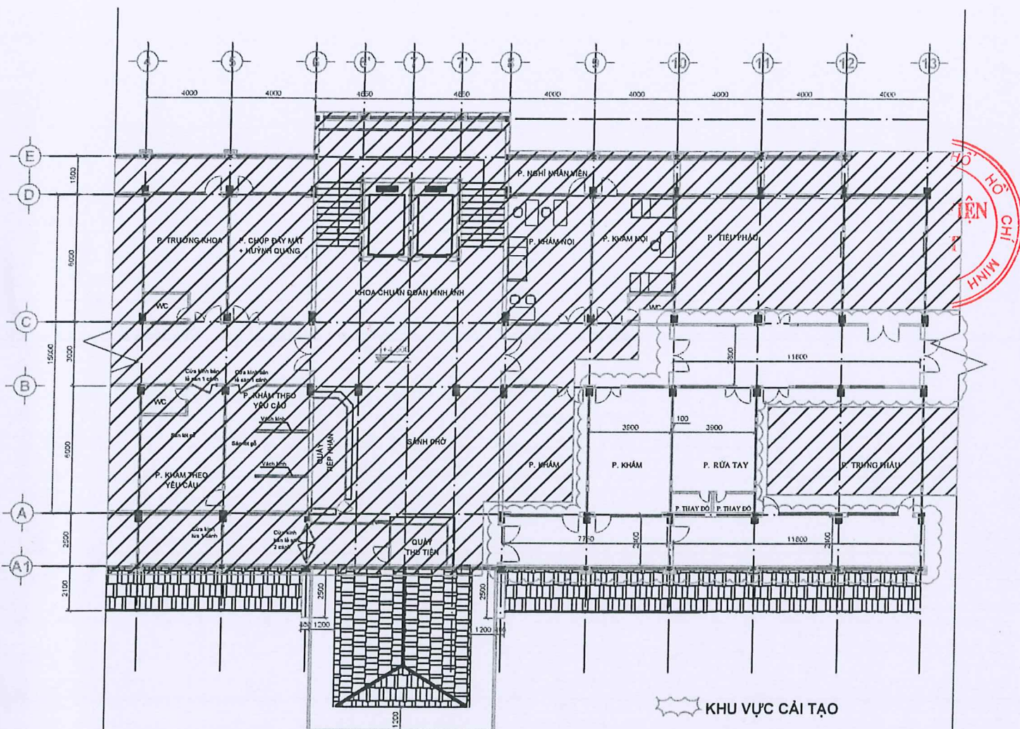
MẶT BẰNG SỬA CHỮA, CẢI TẠO HÀNH LANG VÀ CÁC PHÒNG KHÁM, PHÒNG THAY ĐỒ THUỘC KHU TIÊU PHẪU, TRUNG PHẪU LẦU 1 KHU B
