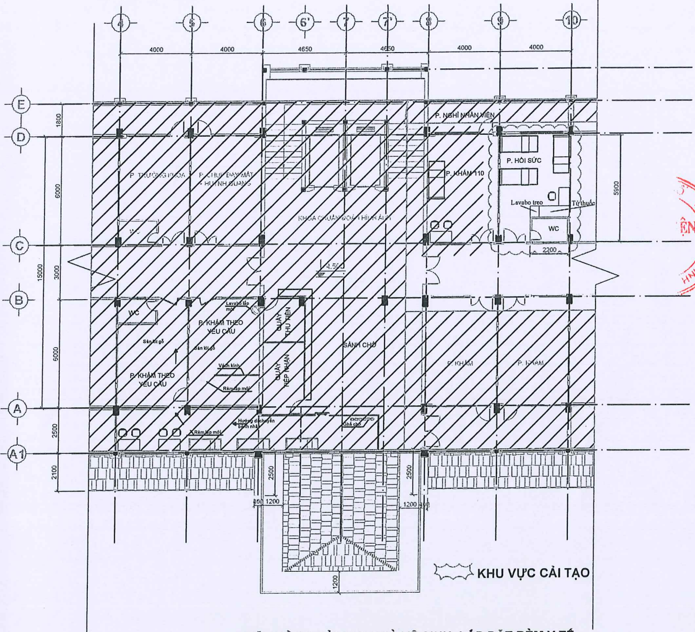
MẶT BẰNG CẢI TẠO NHÀ VỆ SINH, LẮP ĐẶT RÈM Y TẾ PHÒNG HỒI SỨC (PHÒNG KHÁM 112 CŨ) THUỘC KHOA KHÁM
