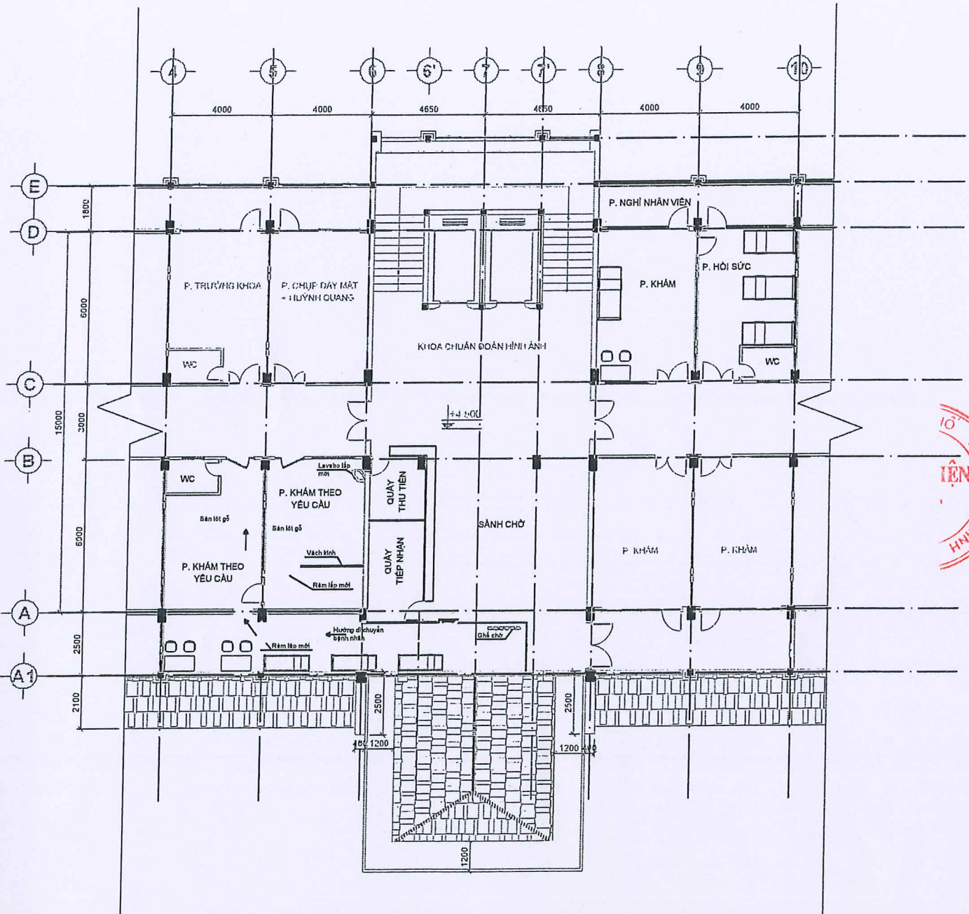
MẶT BẰNG CÀI TẠO TL:1/100
